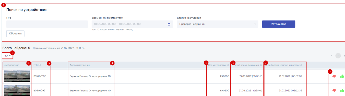
Рисунок 9 – Проверка нарушений.
