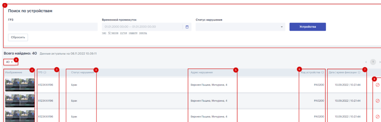
Рисунок 33 – Поиск.
