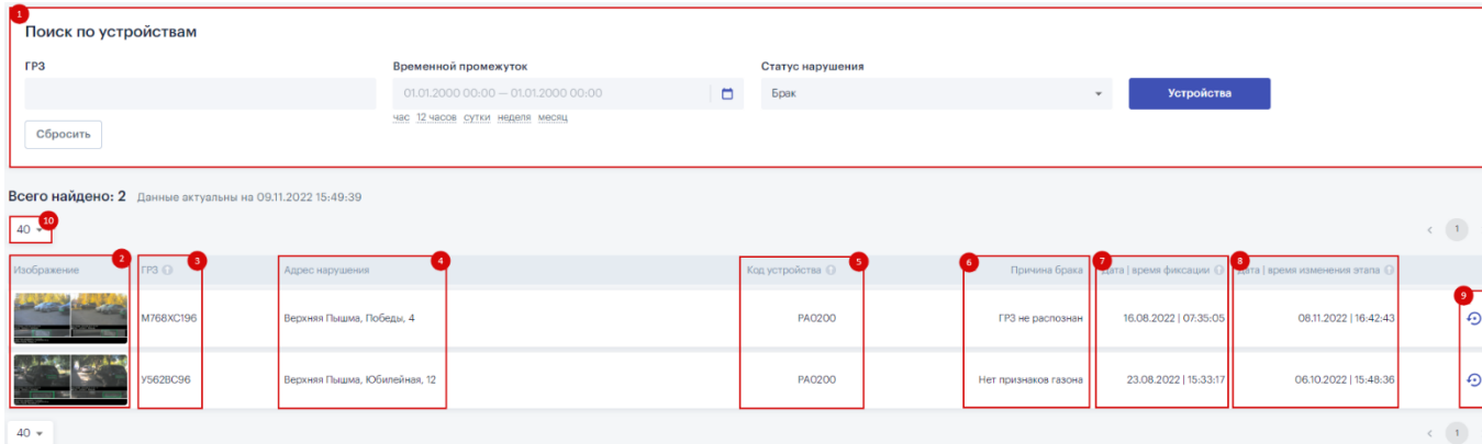
Рисунок 30 – Брак.
