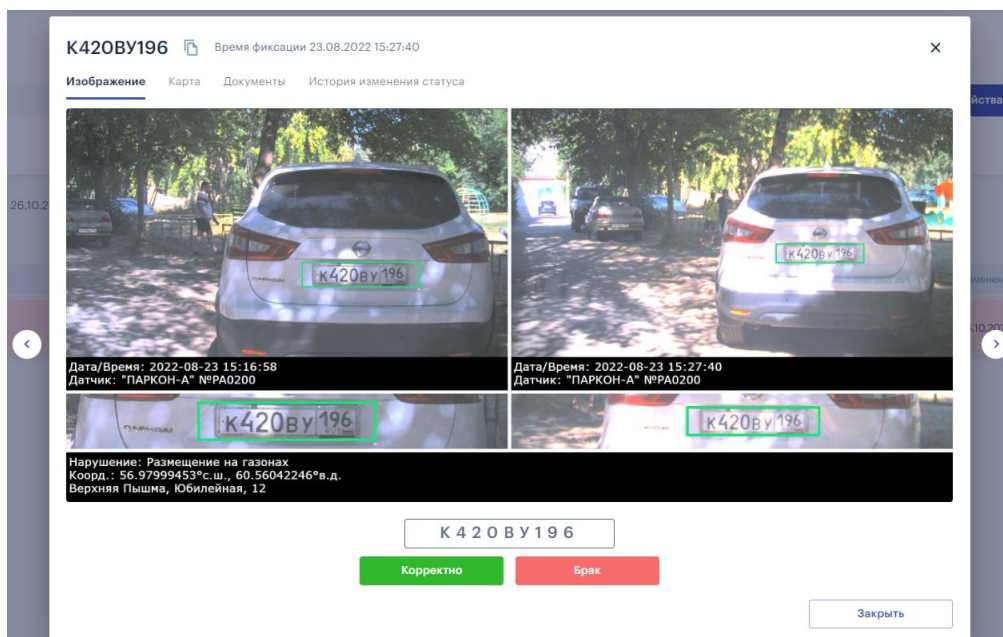
Рисунок 10 – Карточка нарушения.
