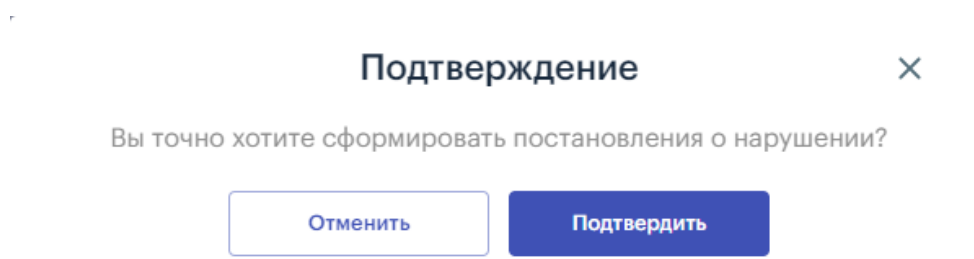
Рисунок 27 – Подтверждение формирования.
