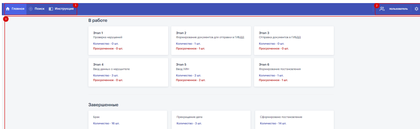
Рисунок 2 – Интерфейс системы.
