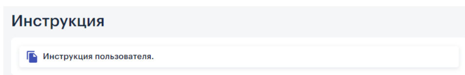
Рисунок 34 – Инструкция.
